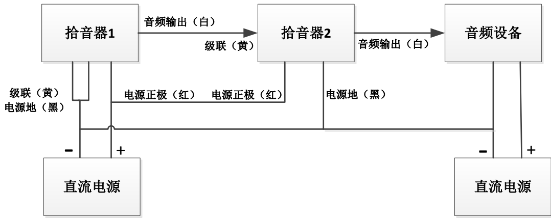
图2-5 级联
