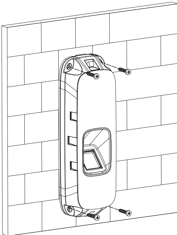
图3-1 安装示意图(1)
