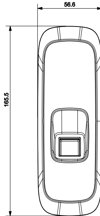
图2-2 结构尺寸 (2)
