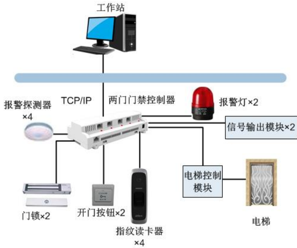
图4-1 系统架构图
