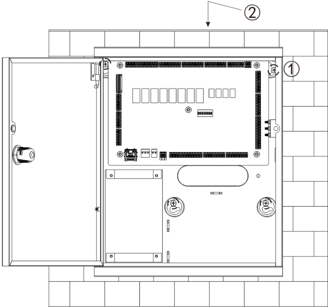
图3-1 安装示意图
