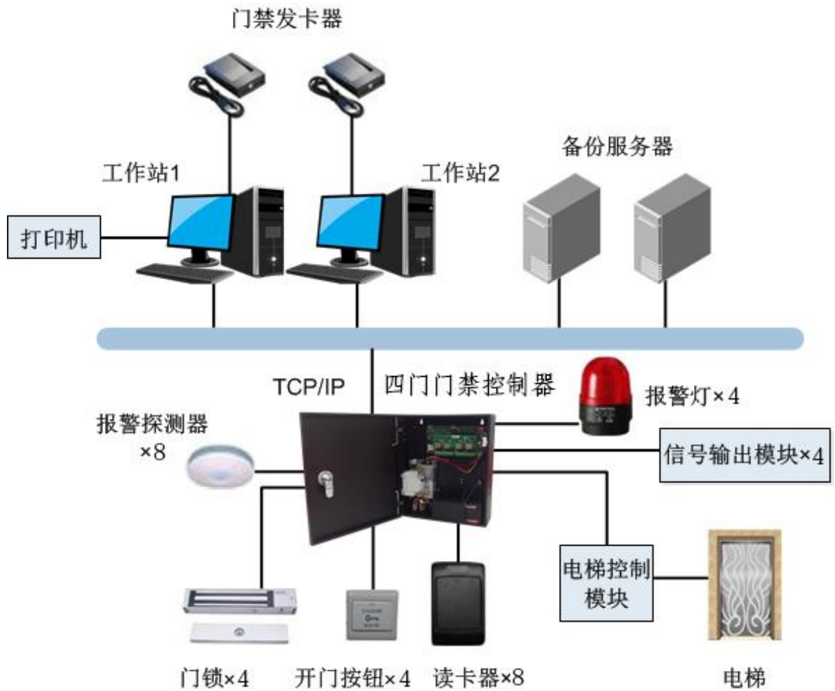
图4-2 系统组网图
