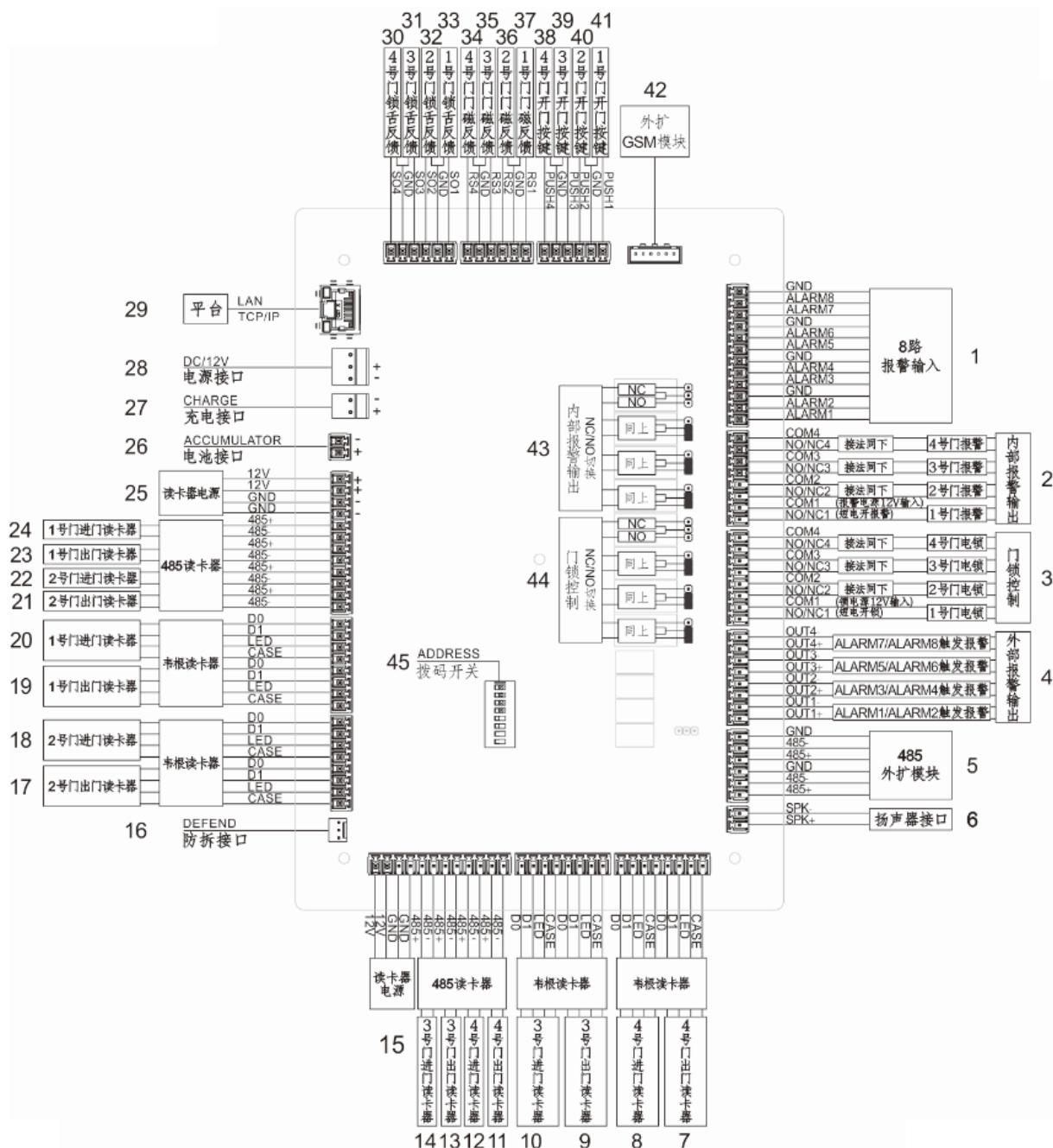
图4-1 接线示意图
