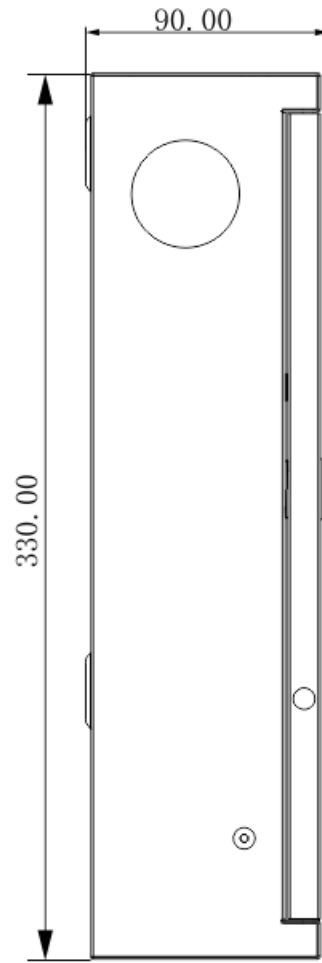
图2-2 外观尺寸 (2)
