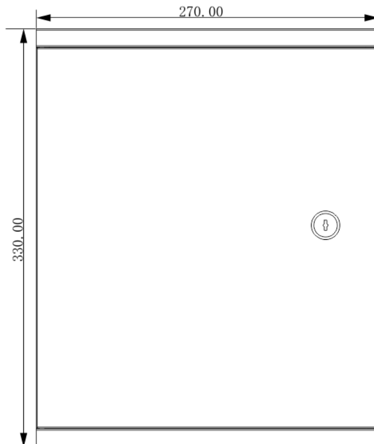
图2-1 外观尺寸（1）
