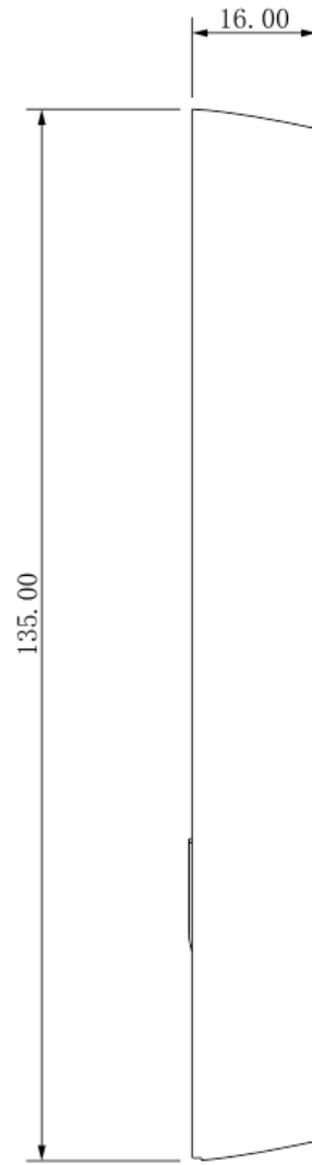
图2-5 结构尺寸
