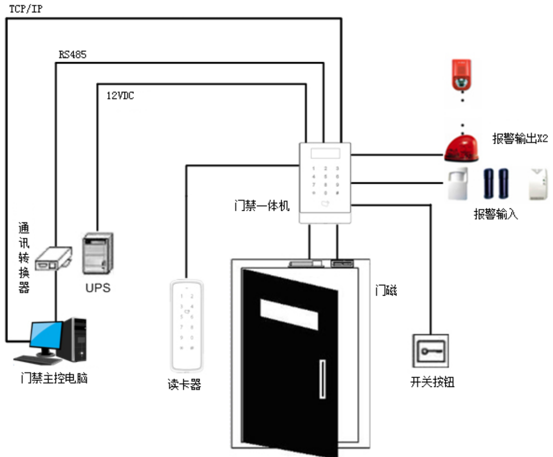
图4-1 系统架构
