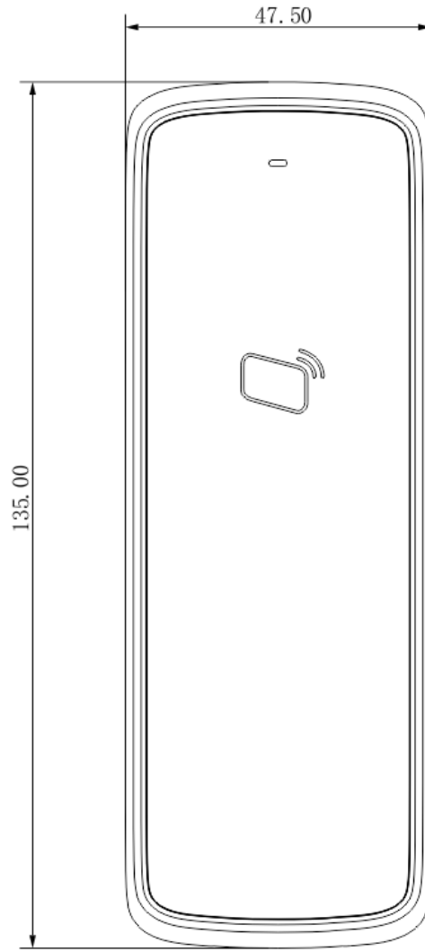
图2-4 结构尺寸（无数字键）
