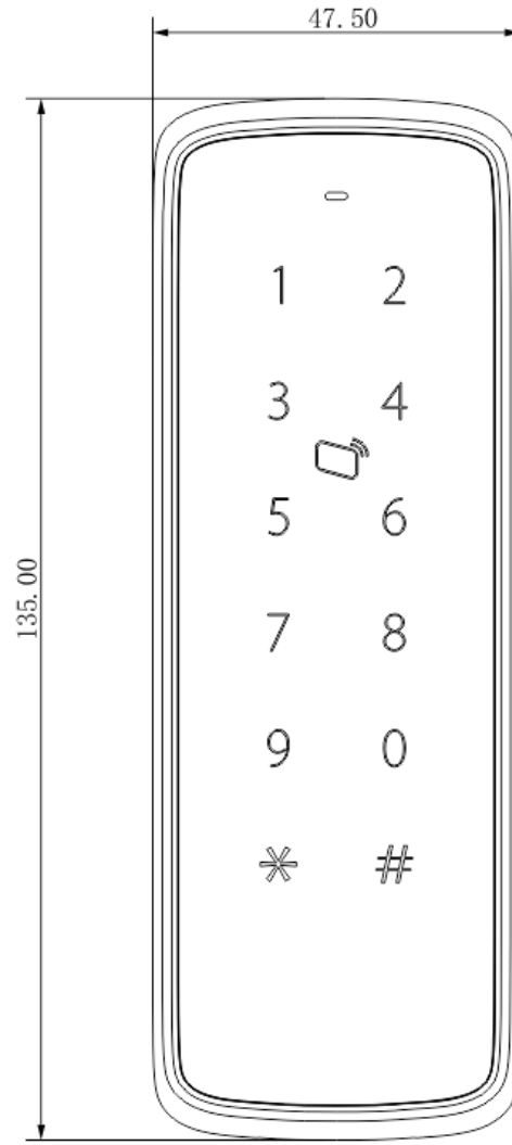
图2-3 结构尺寸（有数字键）
