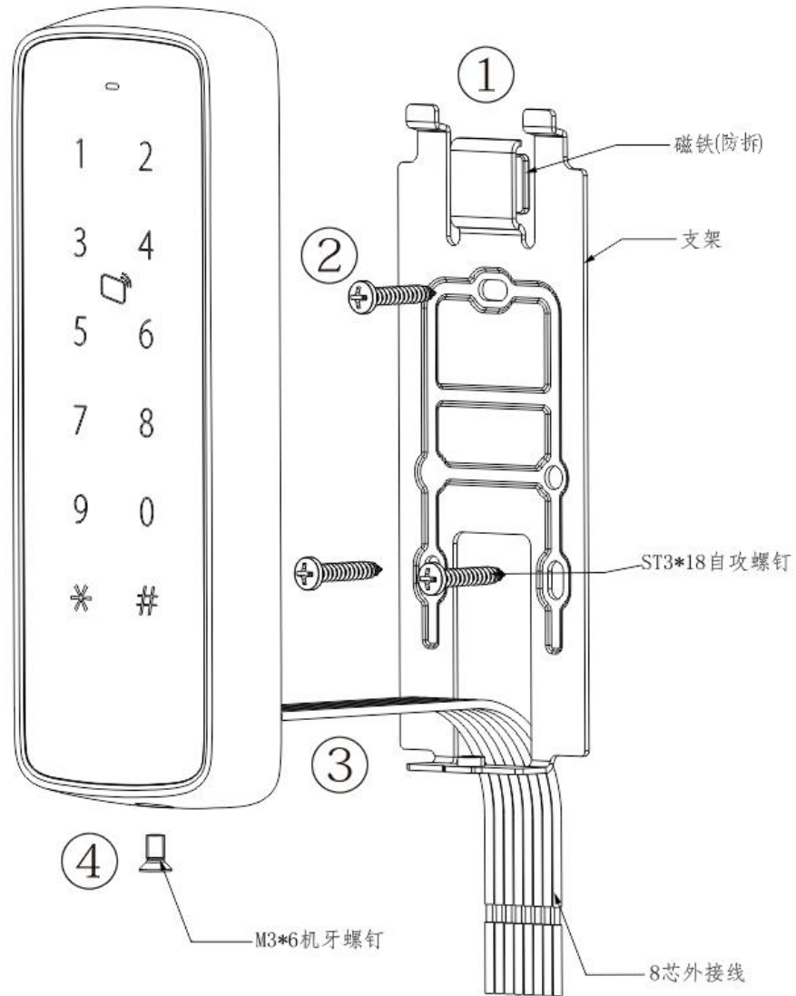
图3-1 安装示意图
