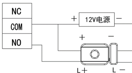
图2-11 磁力锁
