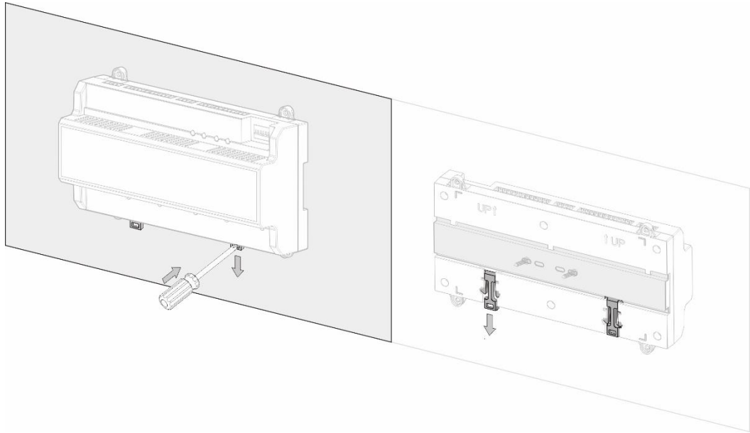
图2-4 拆卸示意图
