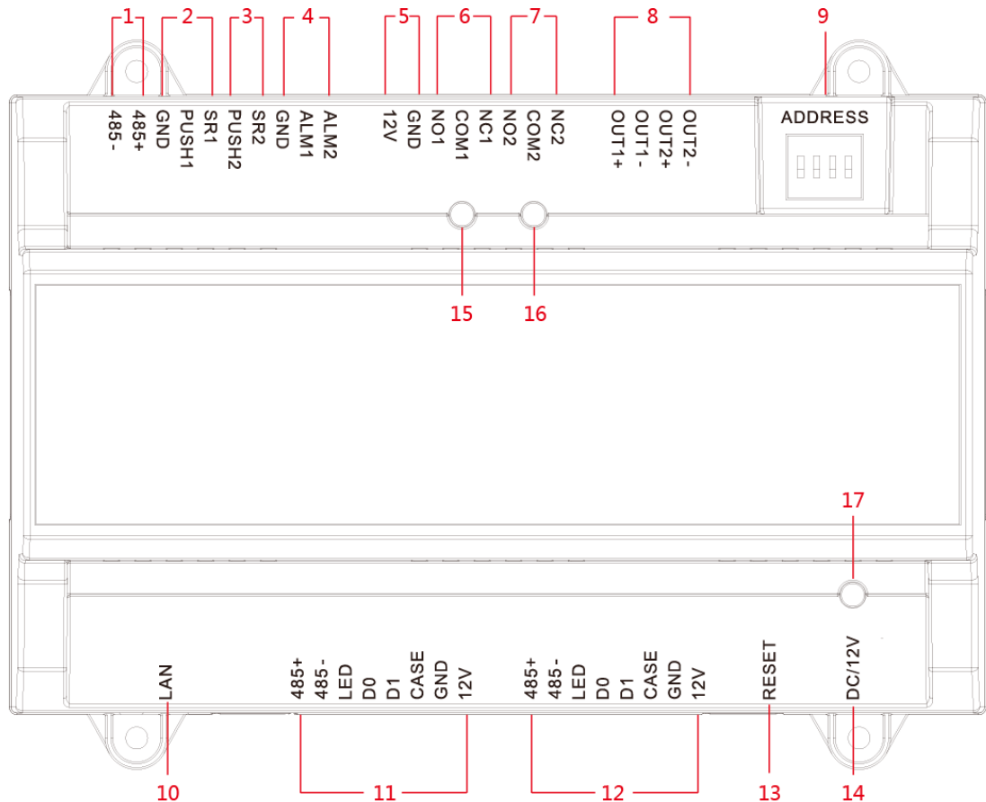
图2-5 接线示意图
