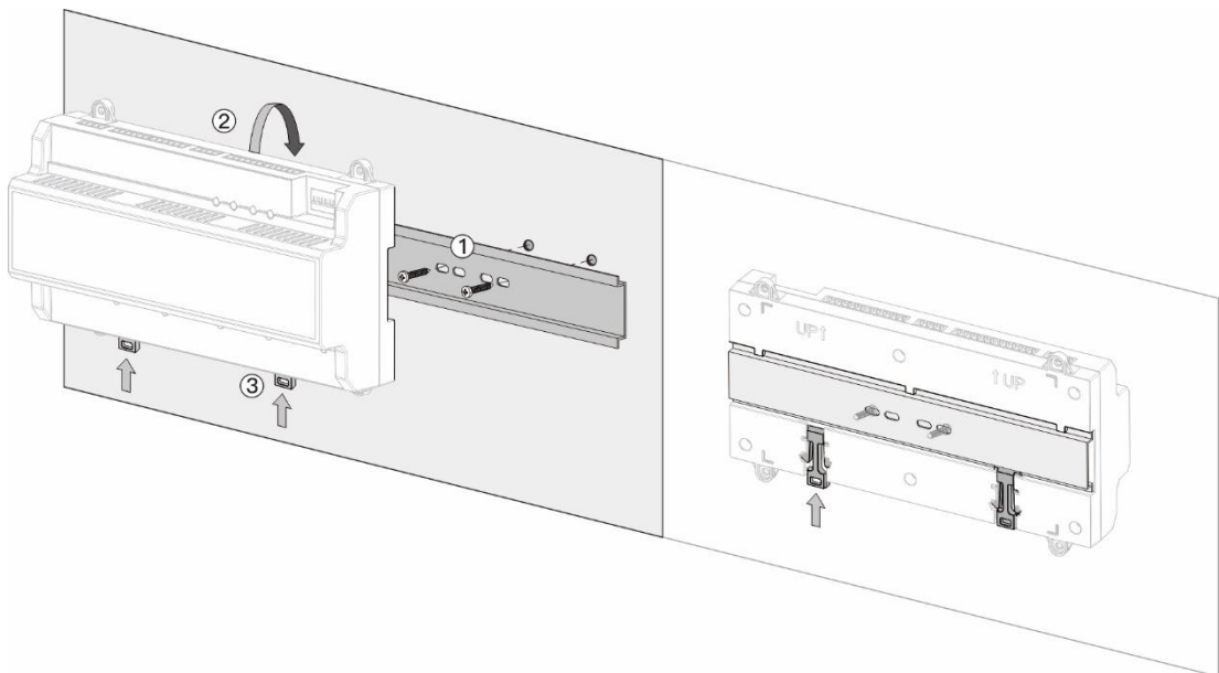
图2-3 安装方式二
