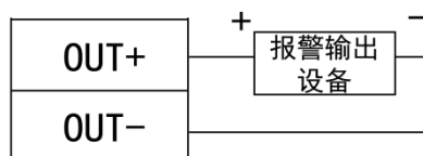
图2-9 报警输出方式二接线图
