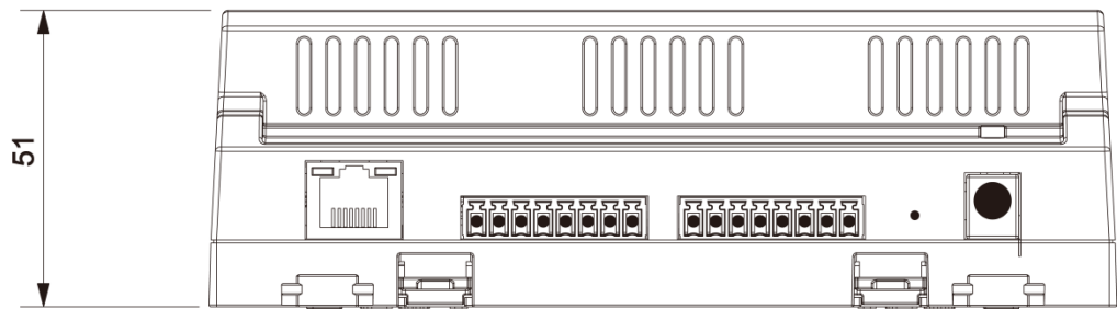
图1-2 外观尺寸 (2) (单位: mm)
