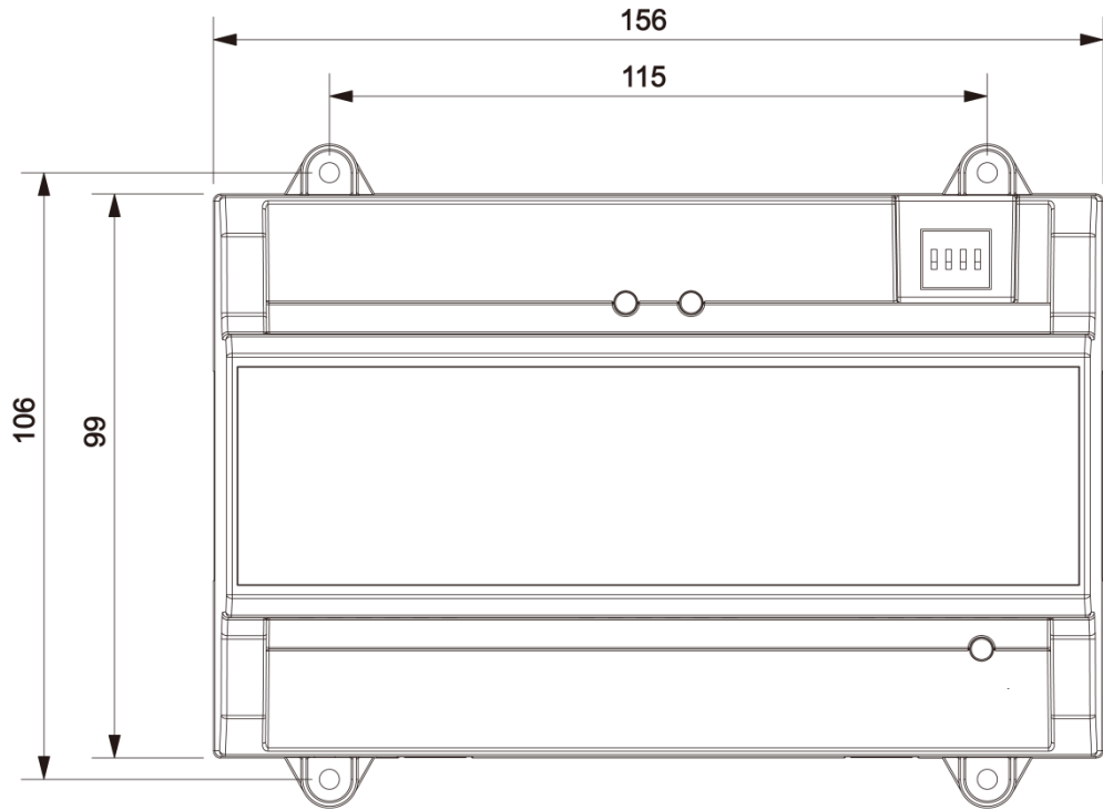
图1-2 外观尺寸 (2) (单位: mm)
