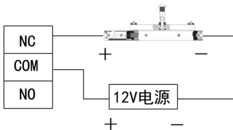
图2-12 电插锁
