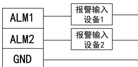
图2-7 外部报警接线图
