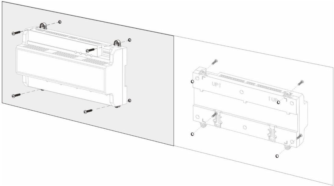
图2-2 安装方式一
