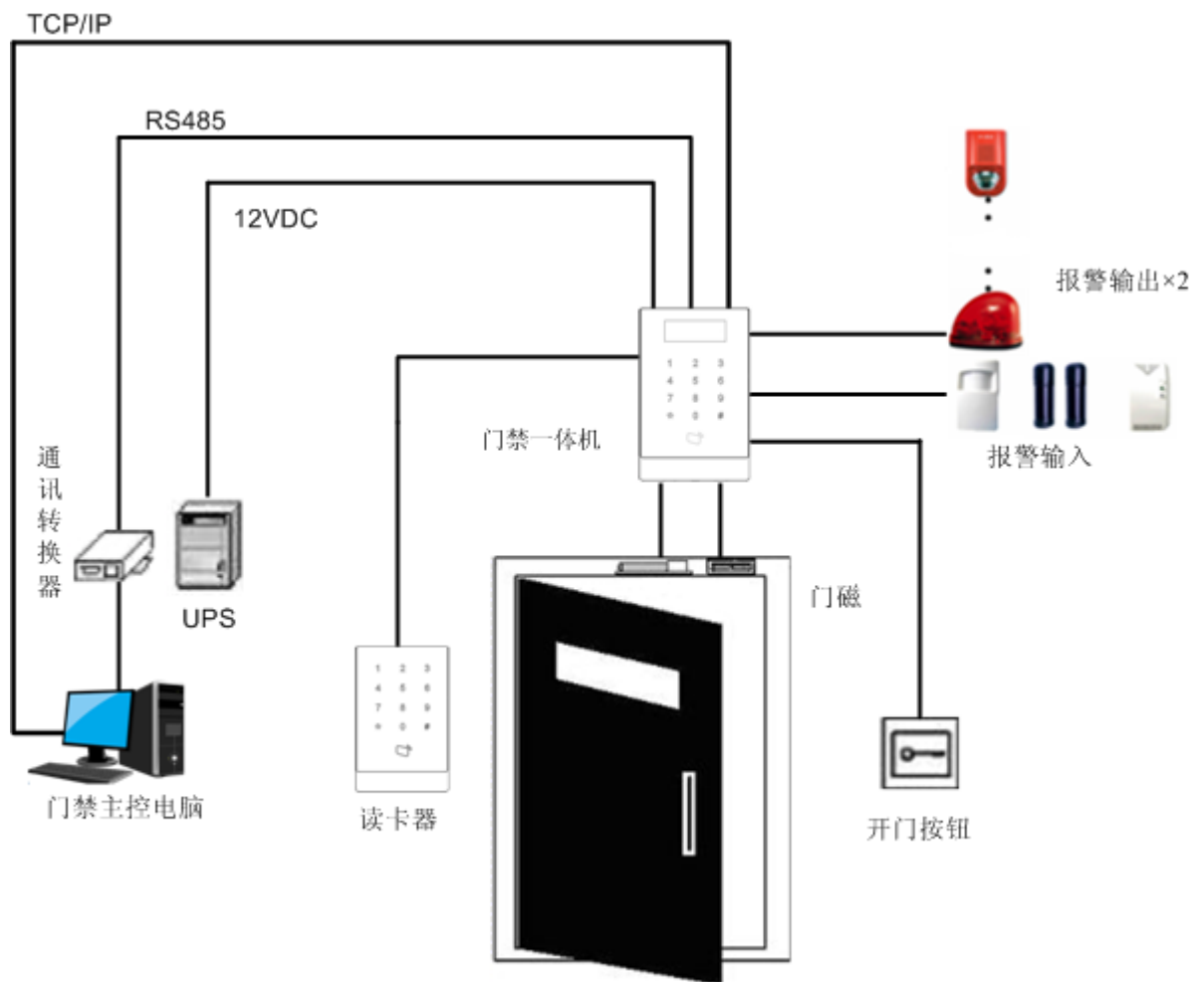
图3-1 系统架构图
