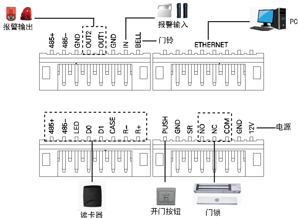
图3-2 接线示意图
