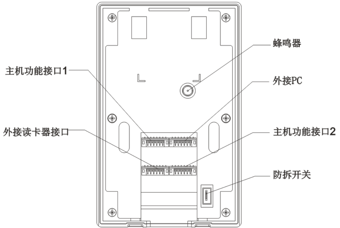
图2-2 设备结构 2
