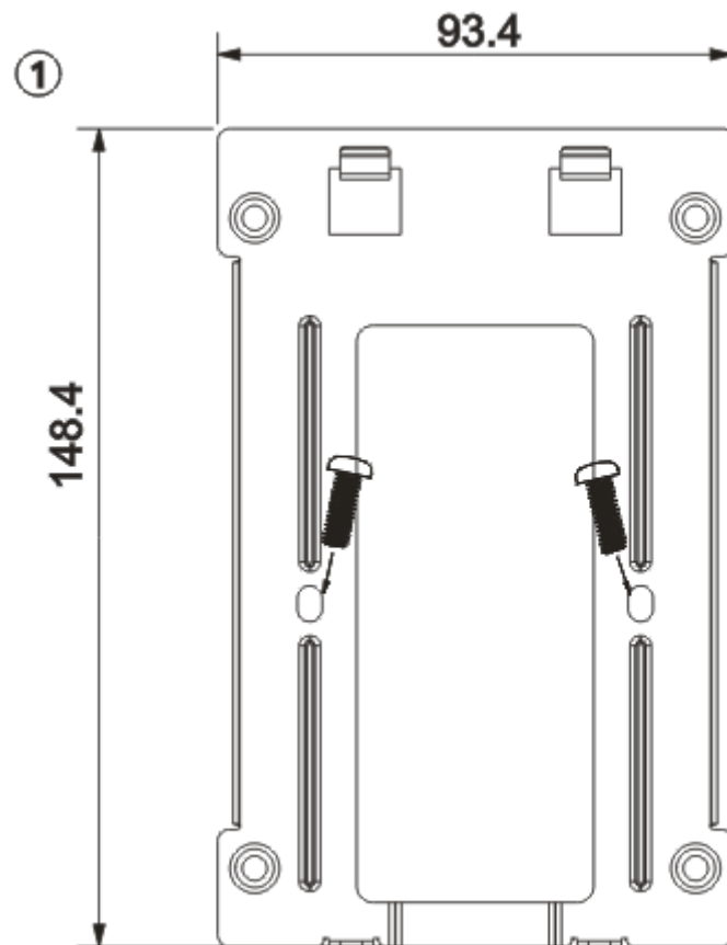
图2-3 设备安装 1
