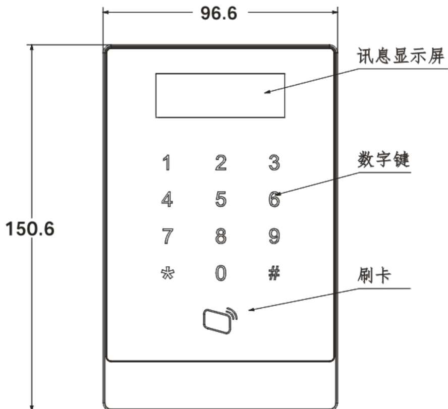
图2-1 设备结构 1
