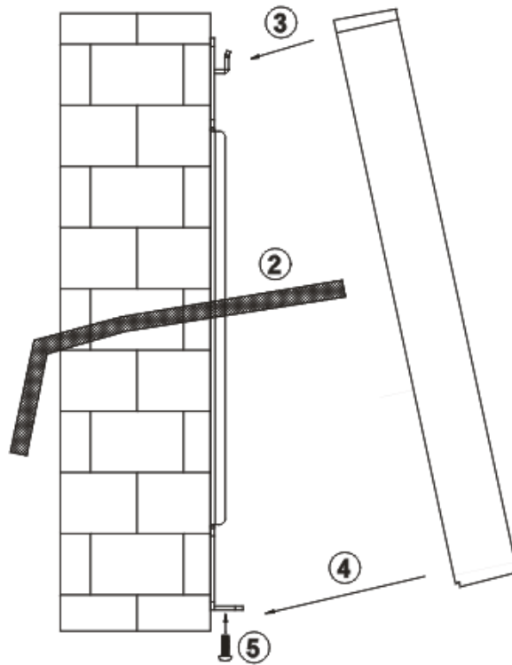
图2-4 设备安装 2
