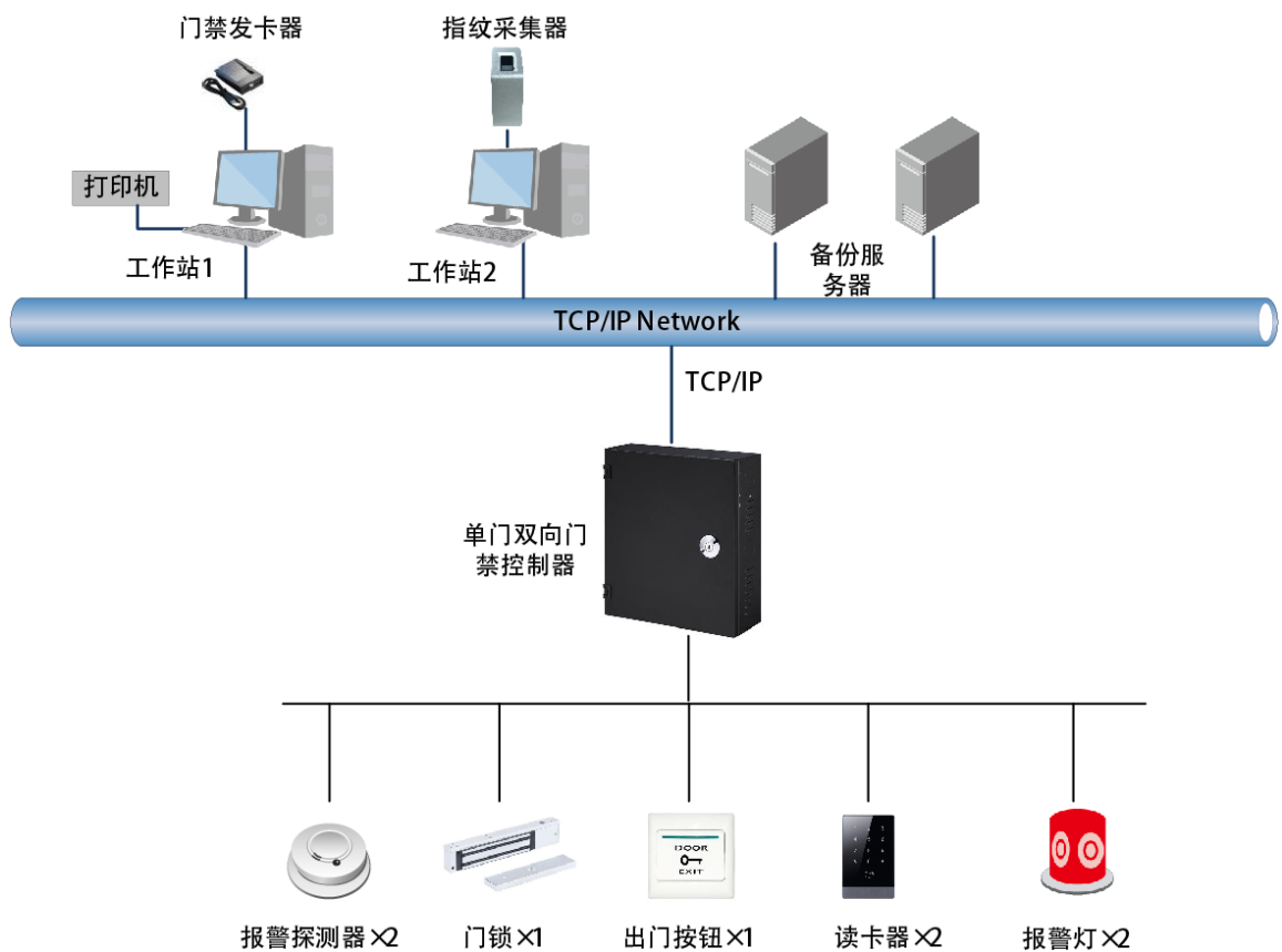
图2-1 系统架构图
