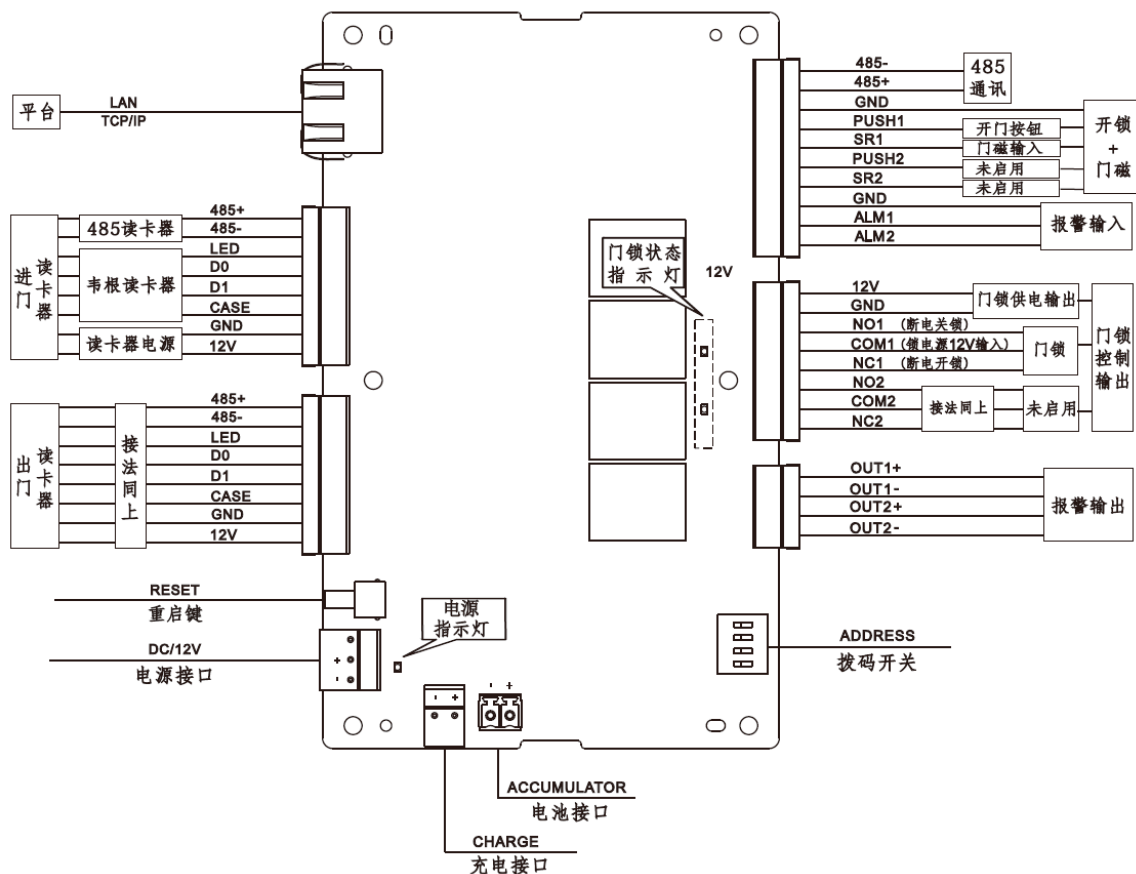
图2-4 接线示意图
