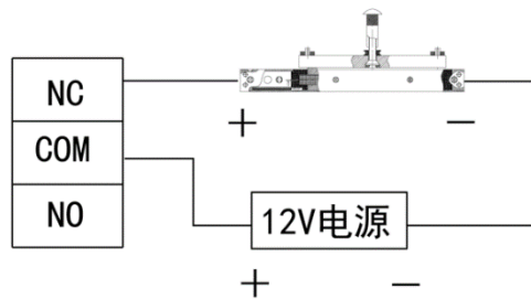
图2-11 电插锁
