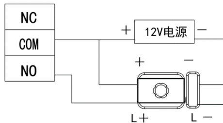
图2-10 磁力锁
