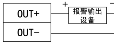
图2-8 报警输出方式二接线图
