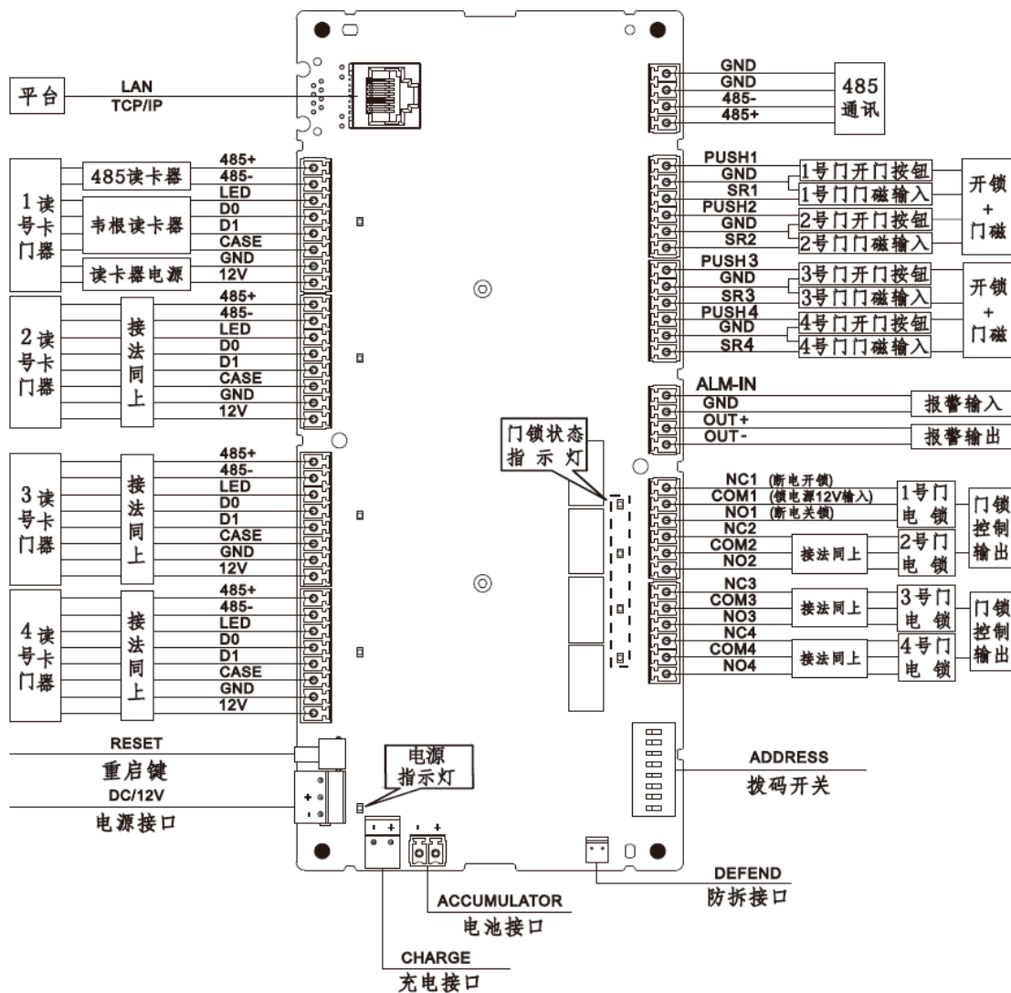
图2-4 接线示意图
