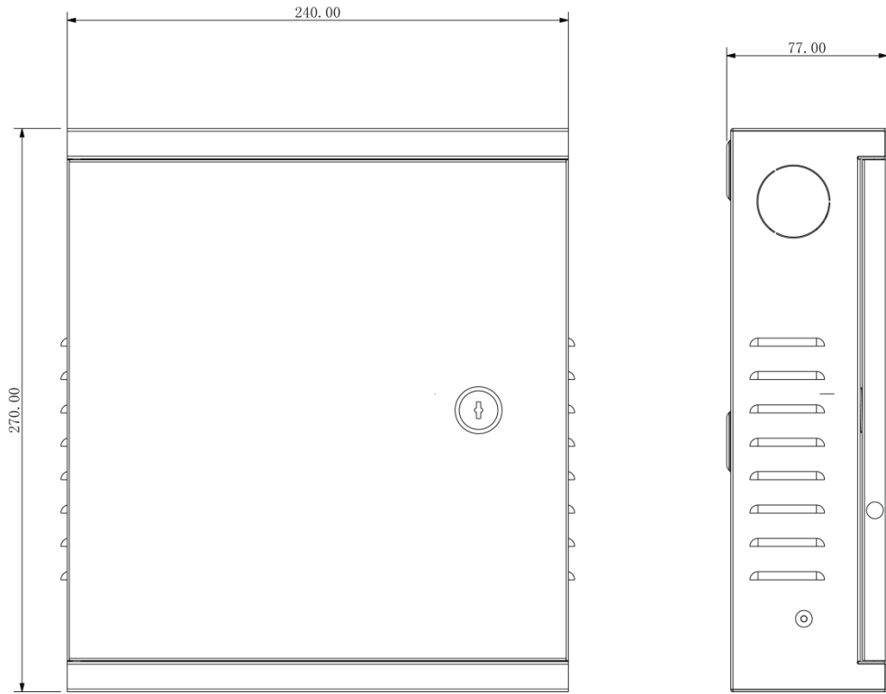
图1-1 外观尺寸 (单位: mm)
