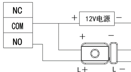
图2-9 电机锁
