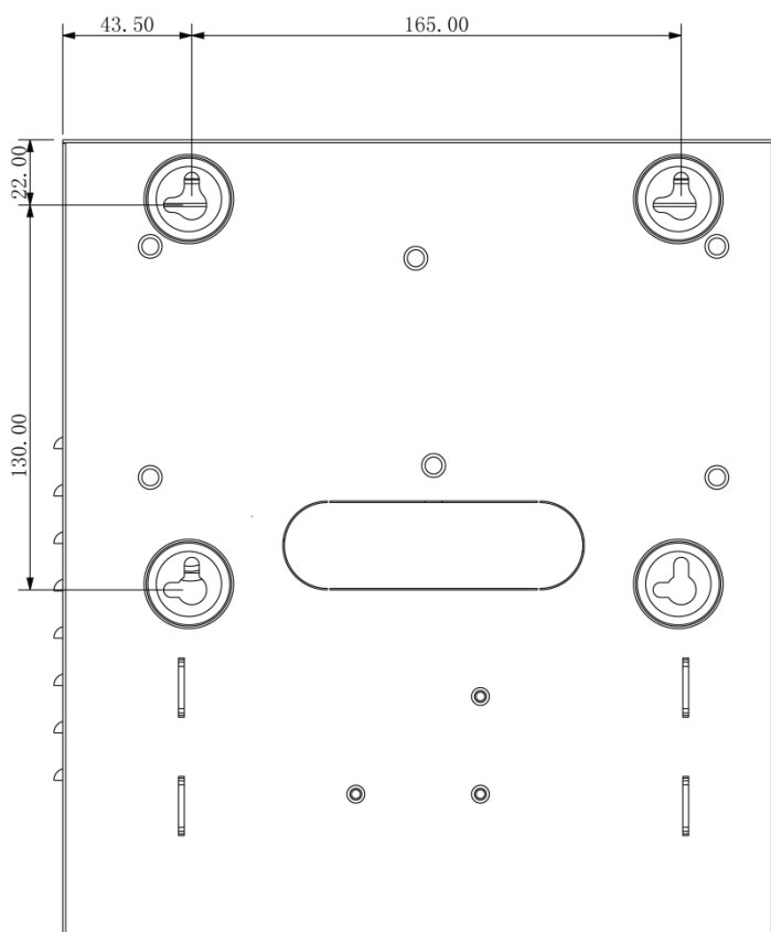
图2-3 安装尺寸图（单位：mm）
