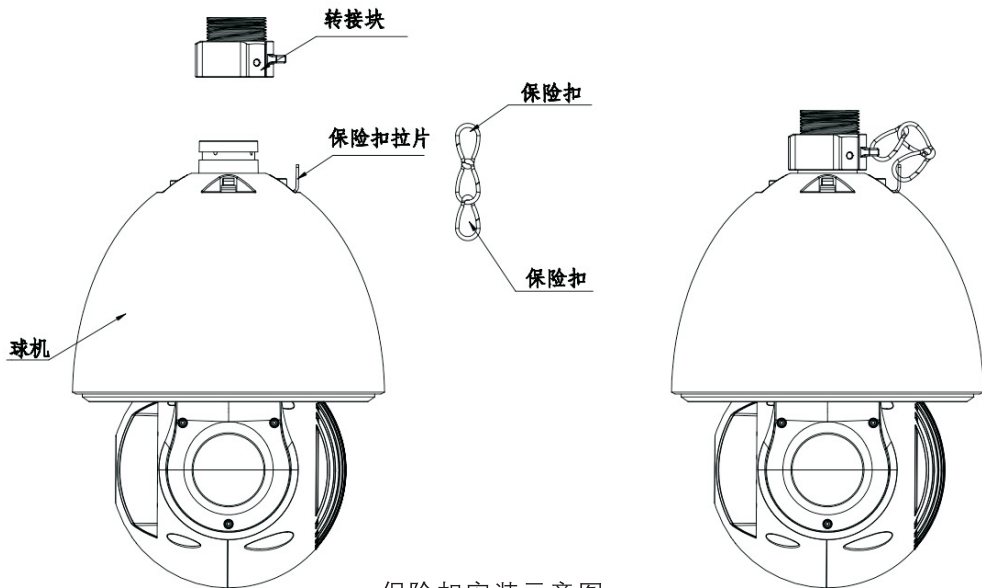
保险扣安装示意图
