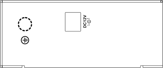
图2-6 上盖意图
