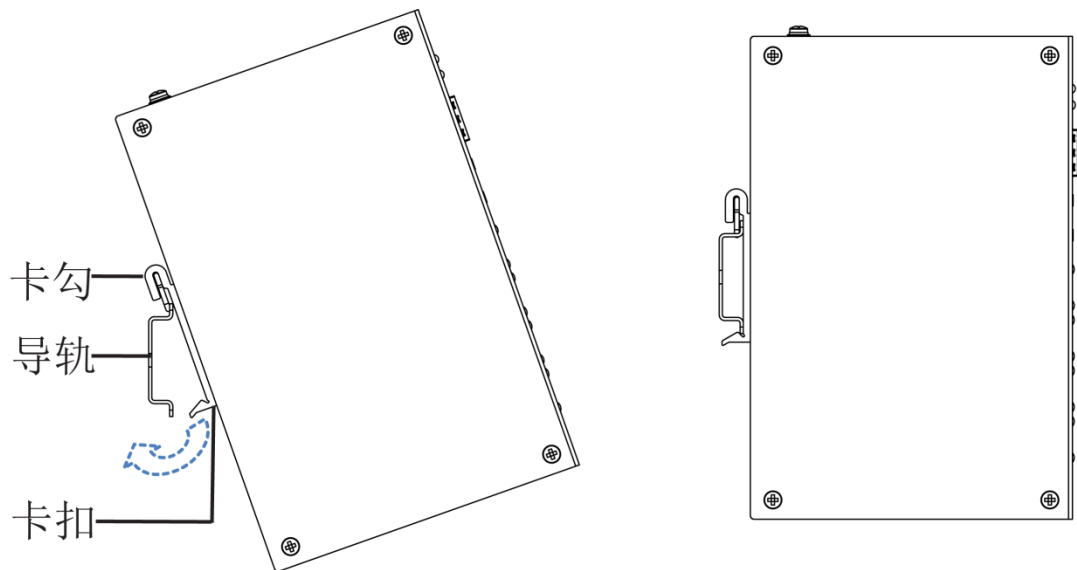
图3-1 导轨装示意图
