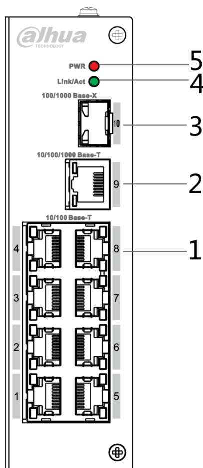
图2-5 前面板意图
