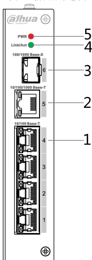
图2-3 前面板示意图
