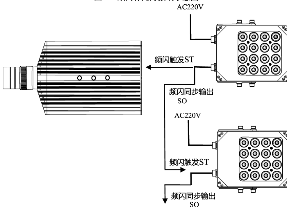
图3-2 频闪补光灯接线示意图
