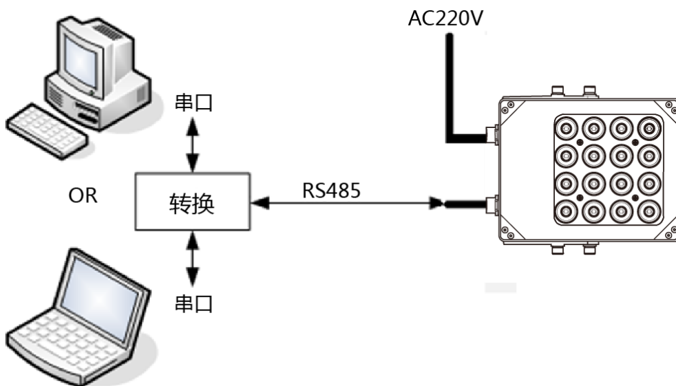
图3-3 RS485 连线说明
