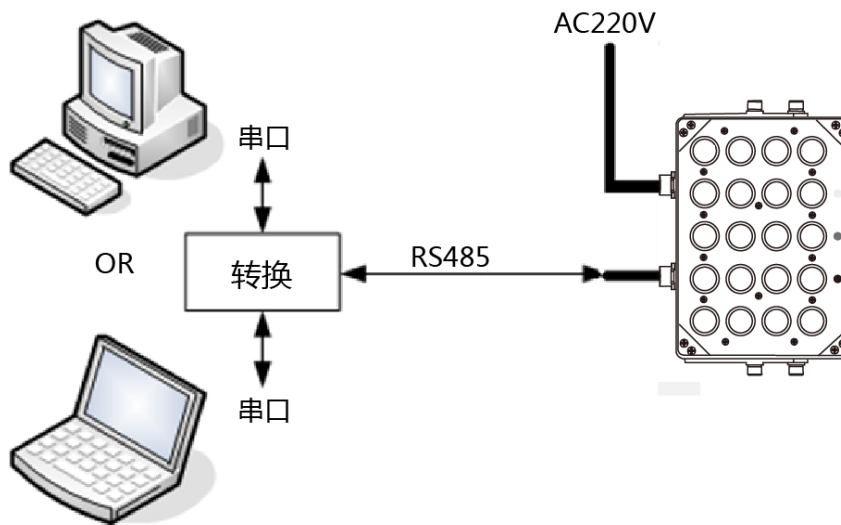
图3-4 RS485 连线示意图
