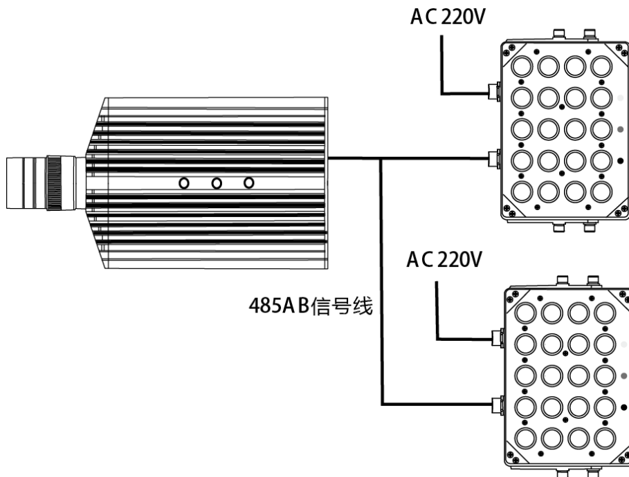
图3-1 补光灯 485 信号线接线示意图
