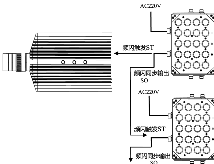
图3-2 频闪补光灯连线示意图
