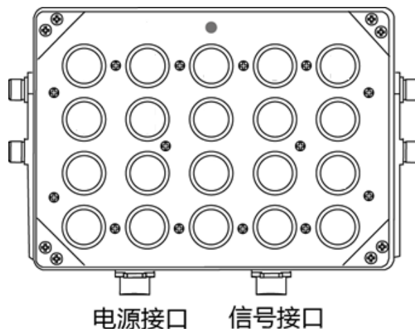
图2-2 灯体前面板
