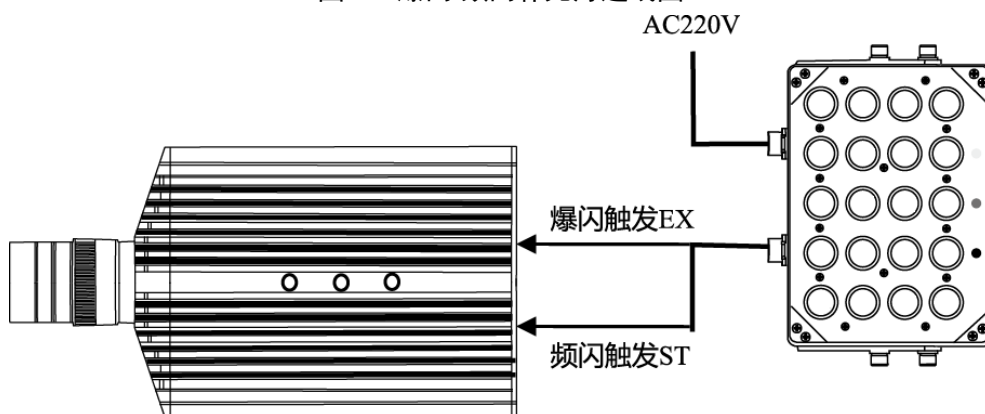
图3-3 爆闪/频闪补光灯连线图
