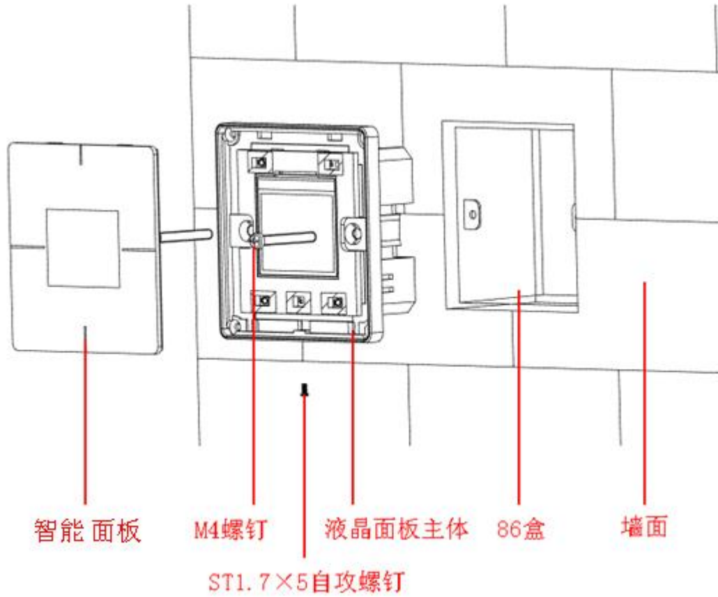
图2-1 安装图
