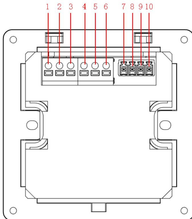
图1-2 设备后面板
