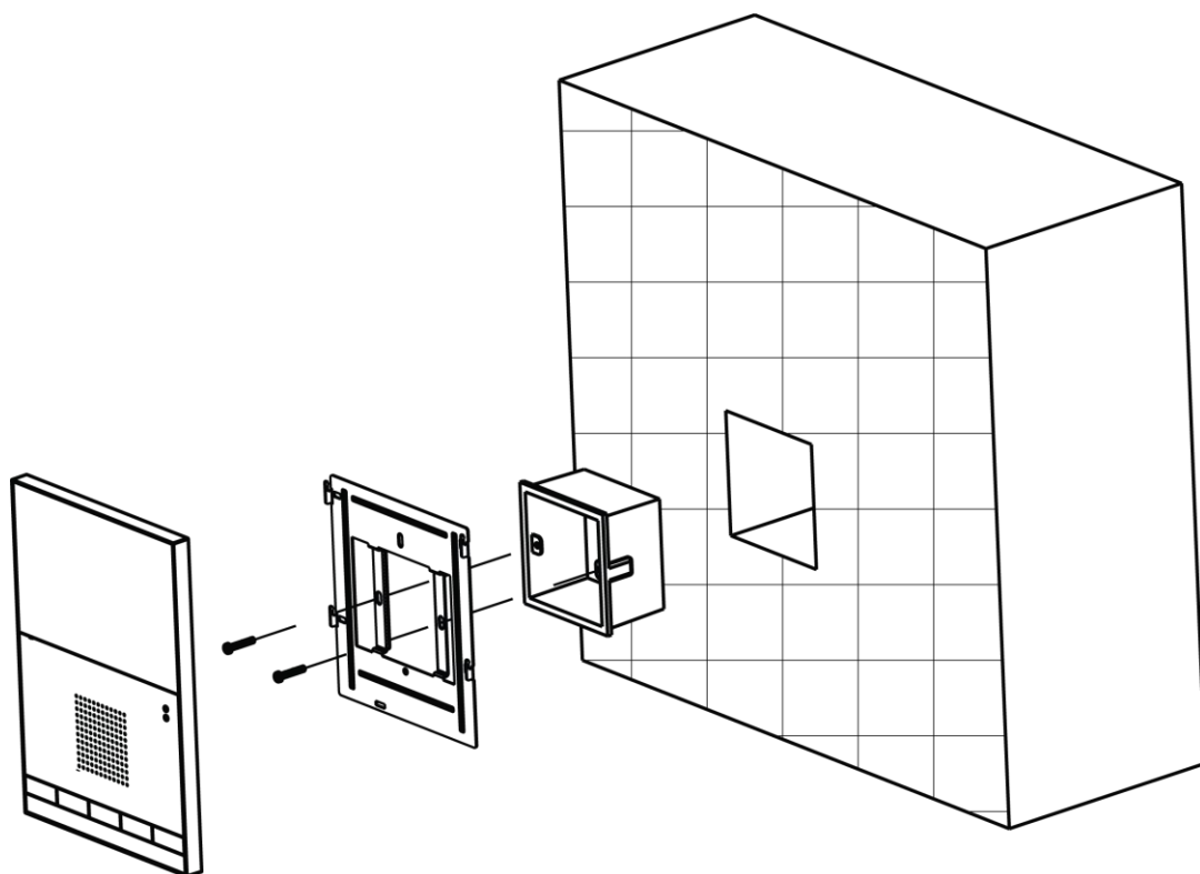
图2-1 安装示意图
