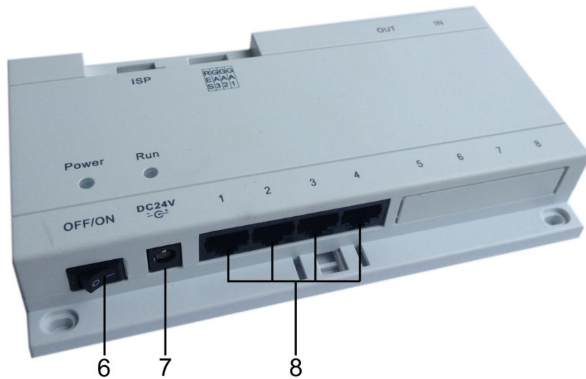
图1-2 4路单元联网分配器正面图
