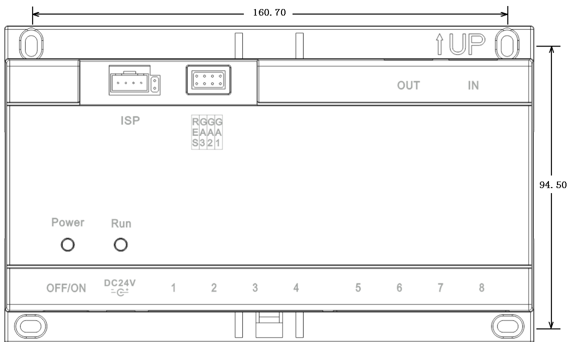
图2-2 安装尺寸图
