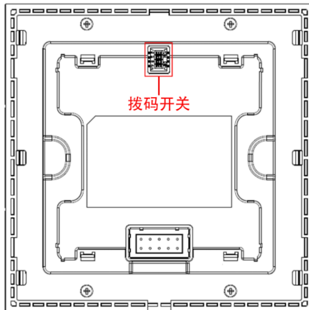
图2-2 前面板背部
