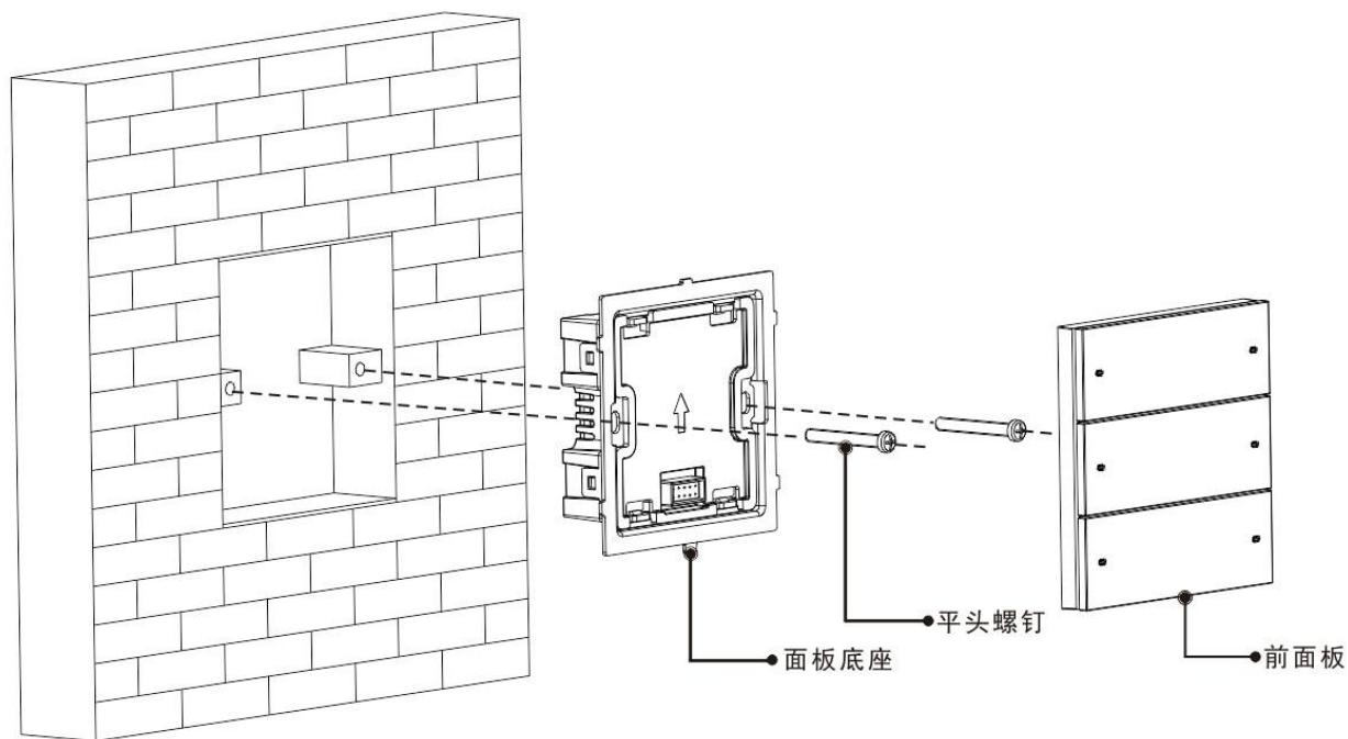
图2-1 安装图
