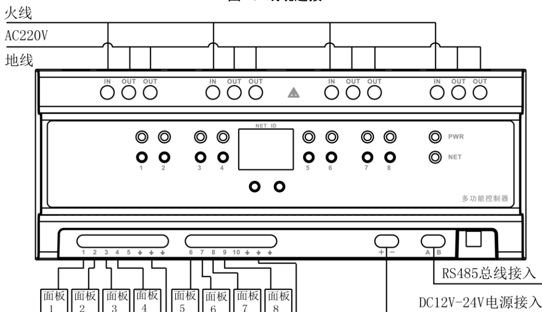
图2-3 线缆连接
