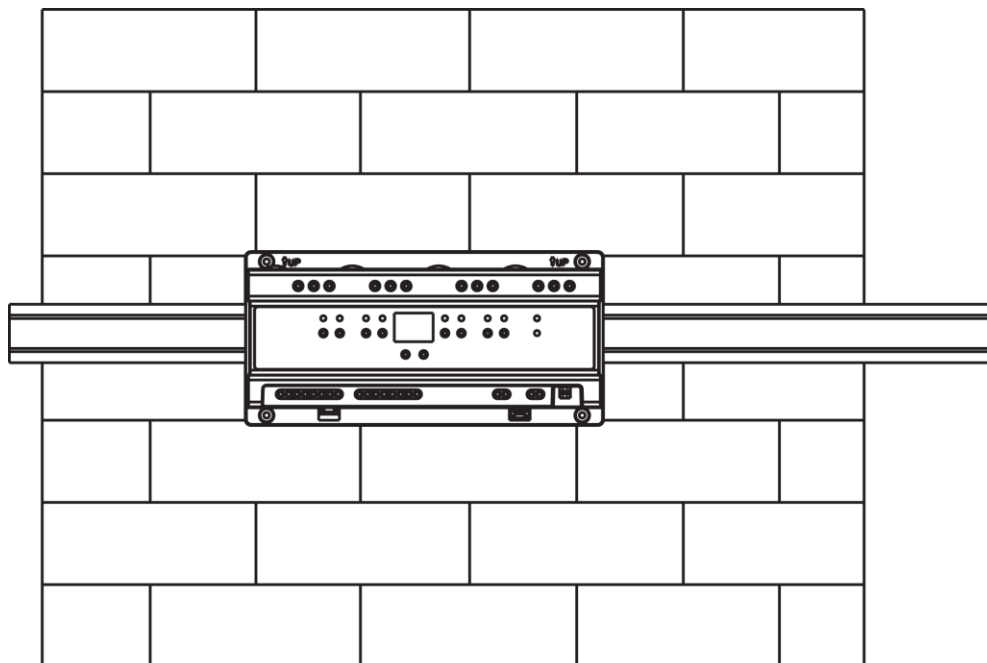
图2-1 安装示意图
