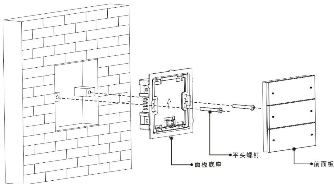
图2-1 安装图
