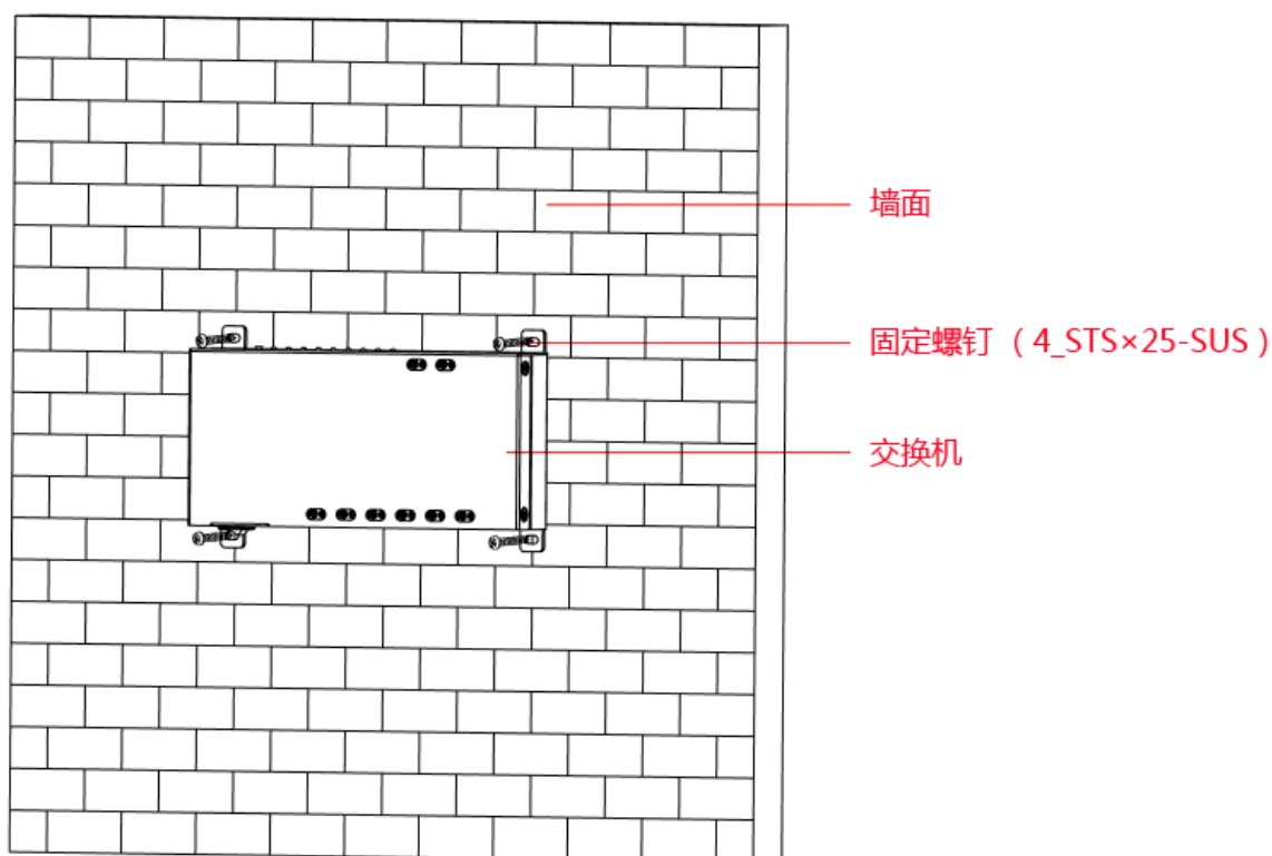
图3-1 壁装（1）
