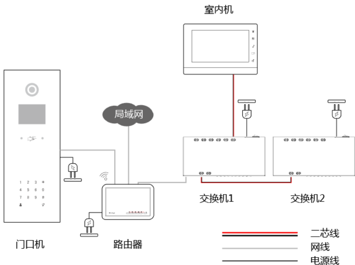
图1-1 组网图
