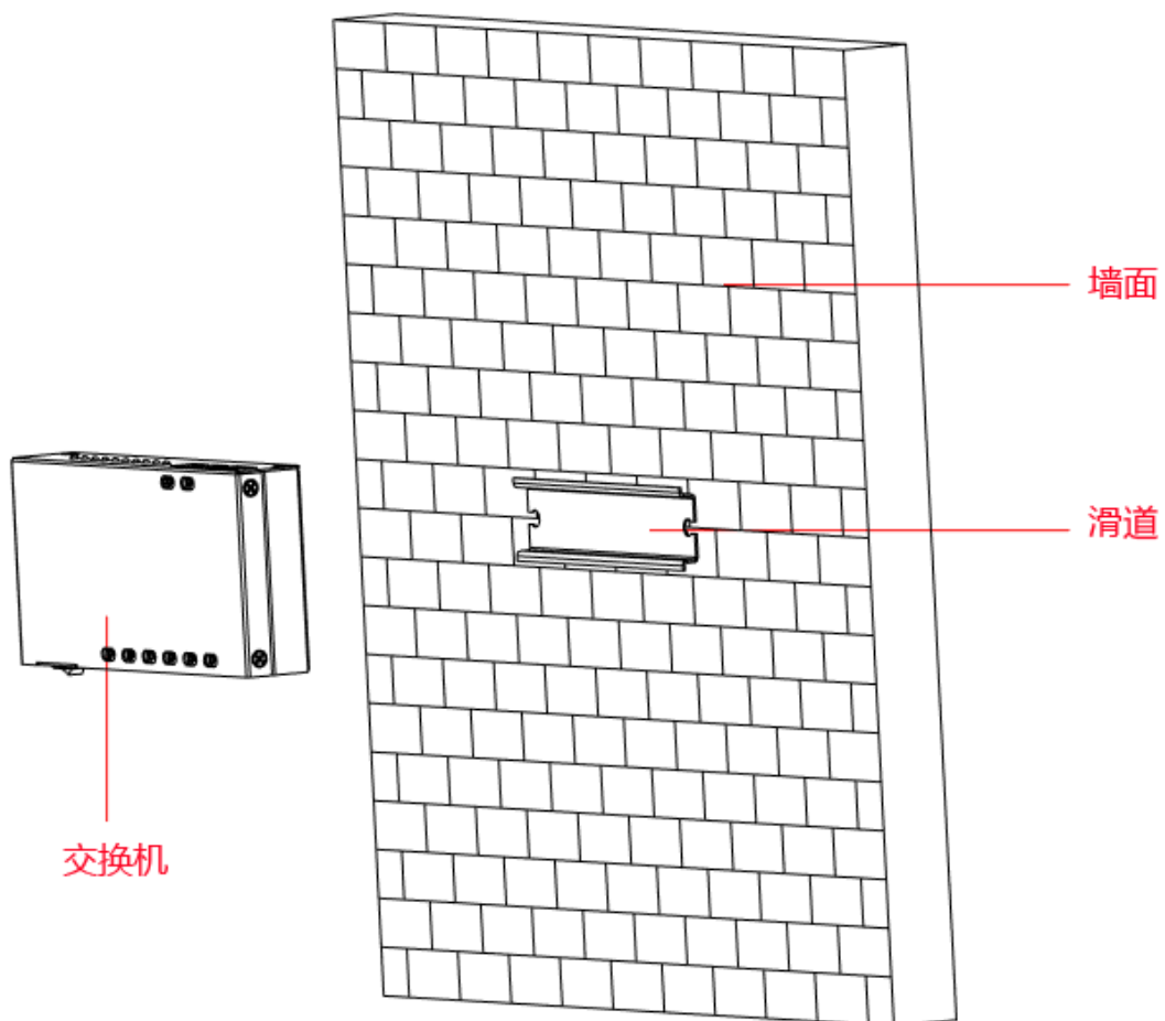
图3-4 壁装 (2)
