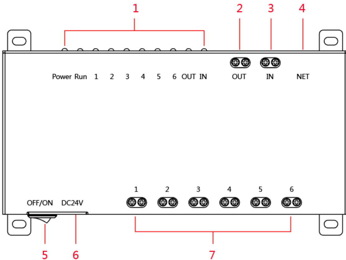
图2-1 设备正面结构图
