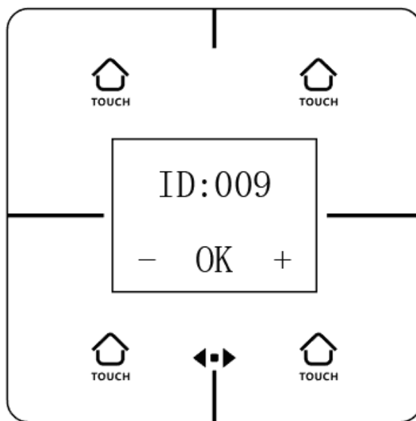
图2-2 ID 设置
