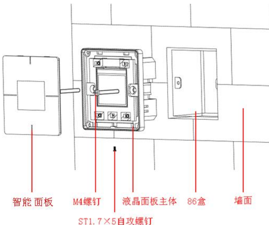
图2-1 安装图
