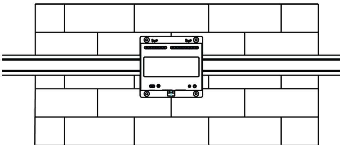
图2-1 导轨安装
