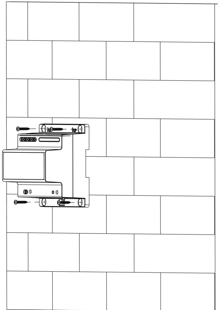
图2-3 墙体安装
