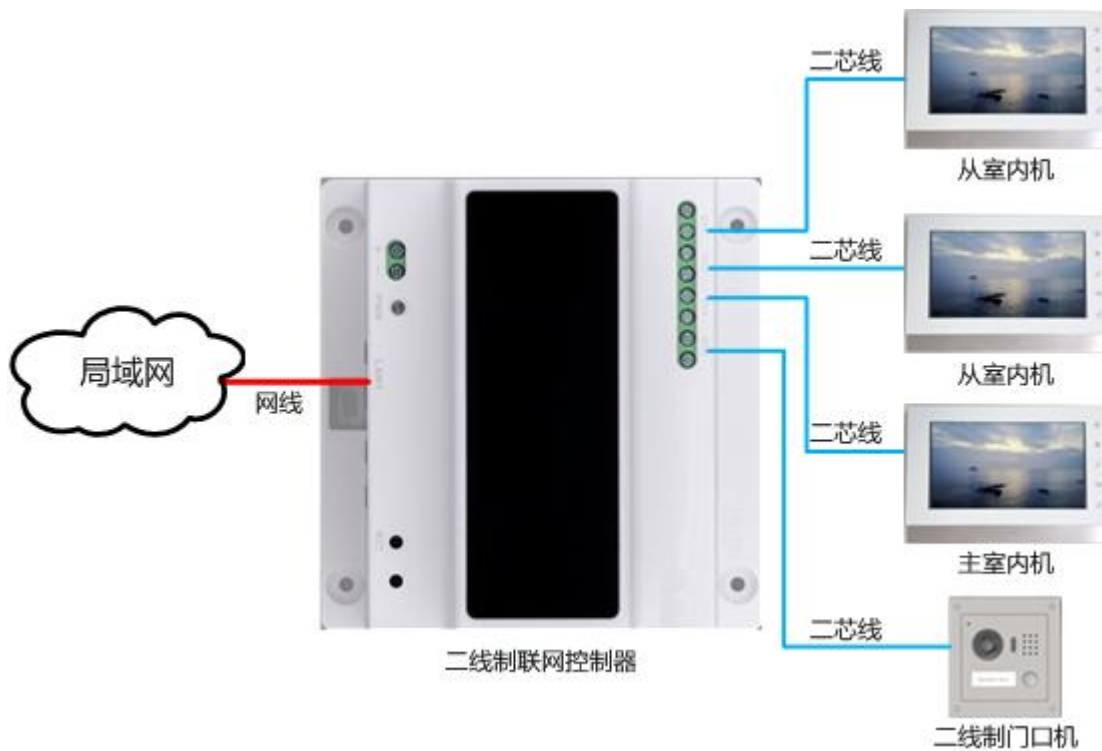
图1-1 组网图
