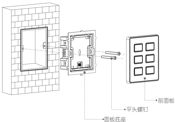
图2-2 安装图
