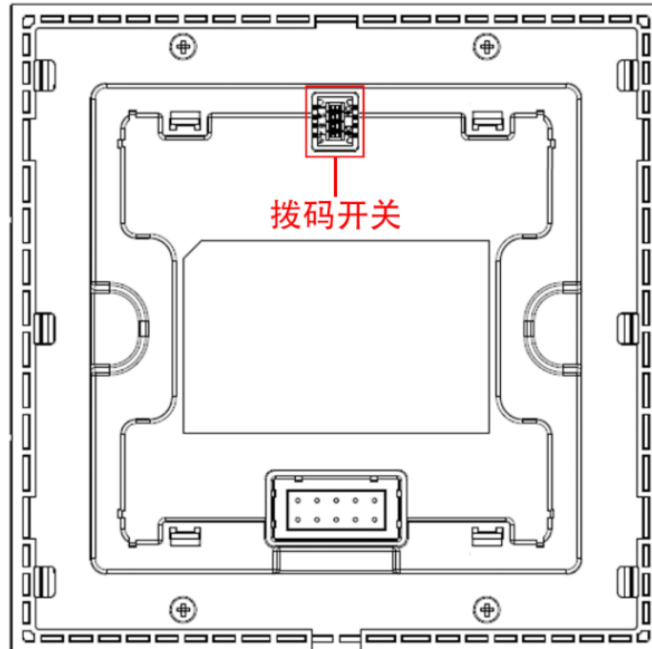
图2-2 前面板背部
