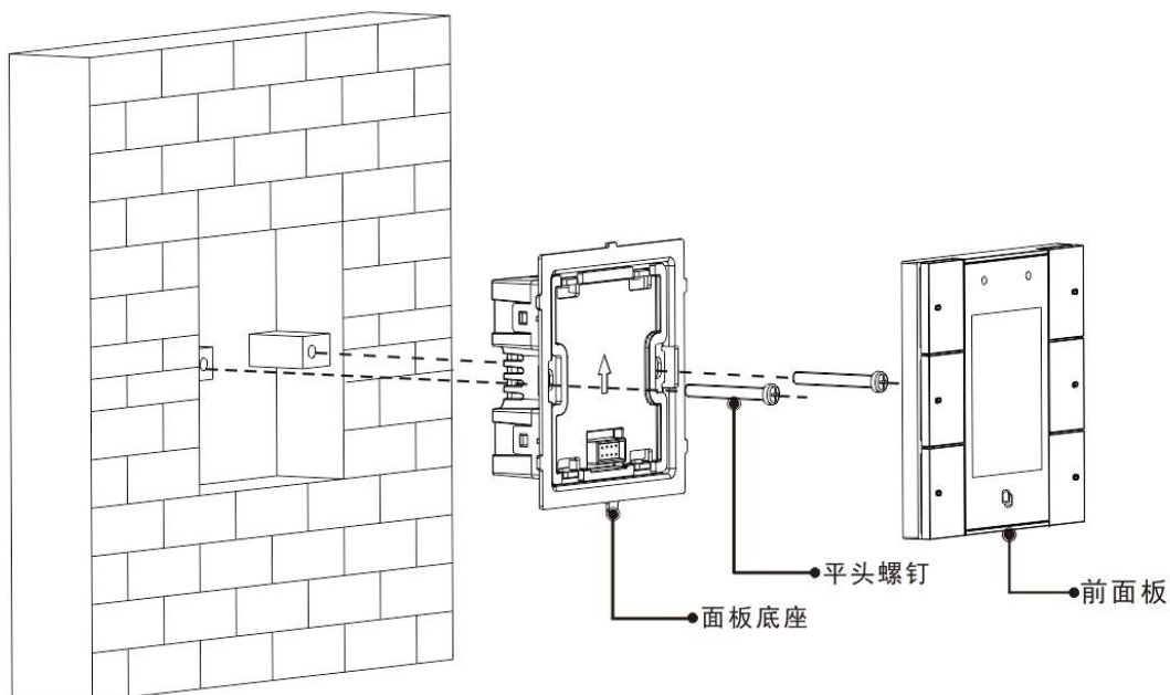
图2-1 安装图
