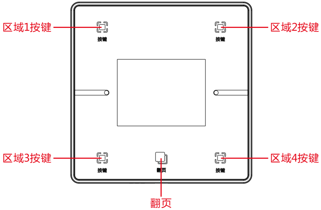
图1-2 触摸按键款前面板
