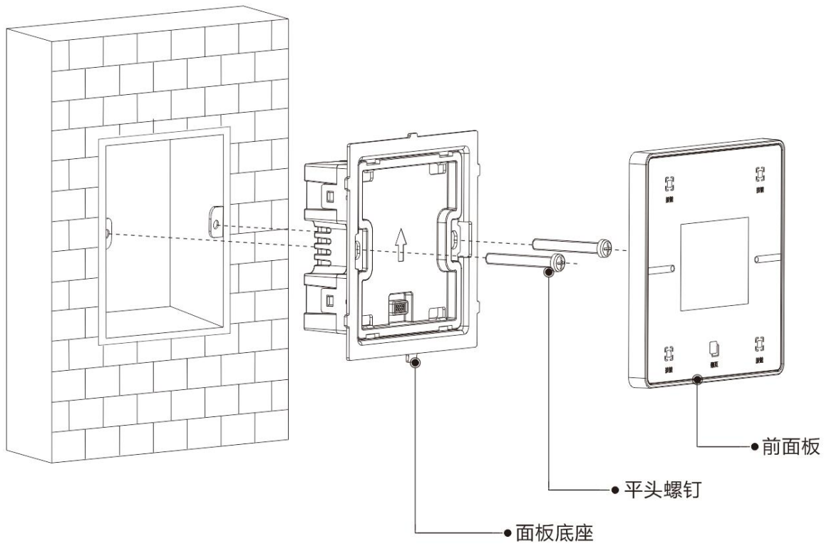
图2-2 安装图
