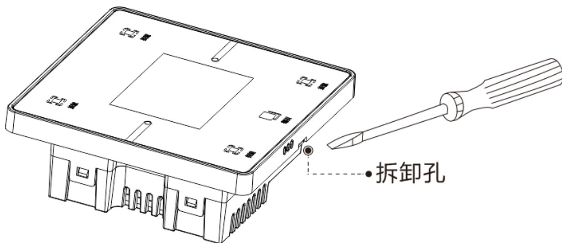
图2-1 拆卸图
